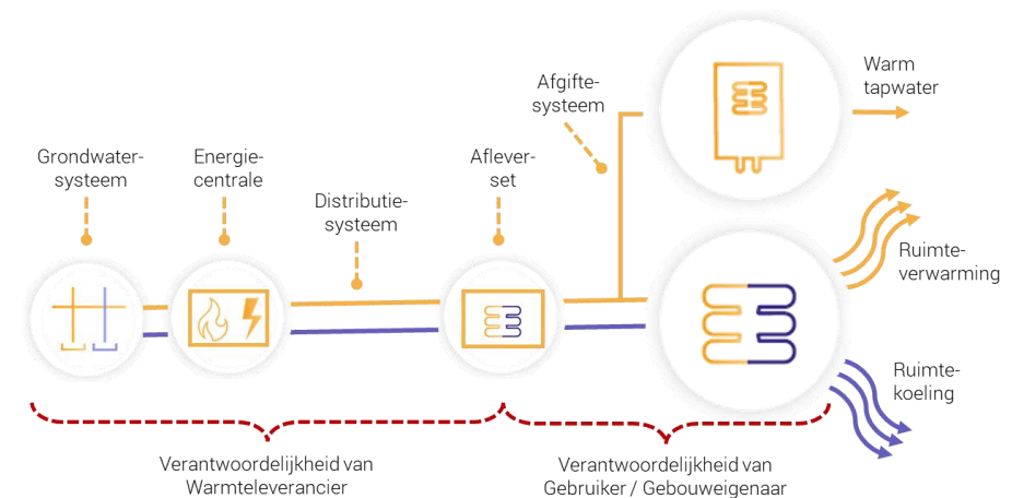
Figuur 11: Schematische afbakening warmteketen en verantwoordelijke partijen. Als een afgiftesysteem in de basis aantoonbaar verkeerd is ontworpen, dan ligt het voor de hand dat de bouw hierop kan worden aangesproken. De gebruiker / gebouweigenaar is verantwoordelijk voor onderhoud van het afgiftesysteem.
